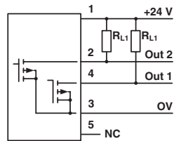
2 X NPN
